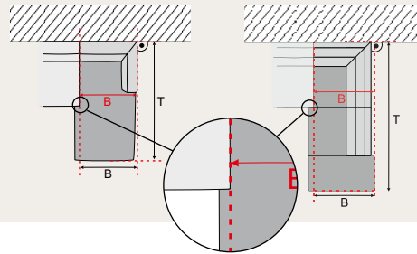
Beispiele: Anstellteile Longchairs und Ecksofas Achtung: Hier wird die tatsächliche Anstellbreite angegeben! Abweichungen vermerken wir in den betreffenden Modellblättern/Technischen Informationen.
